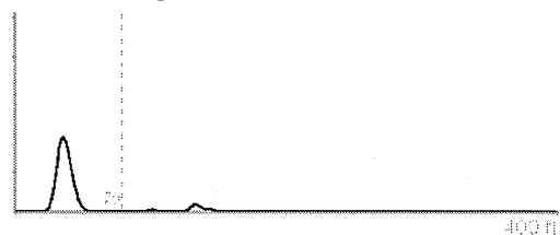
PLT Histogram
